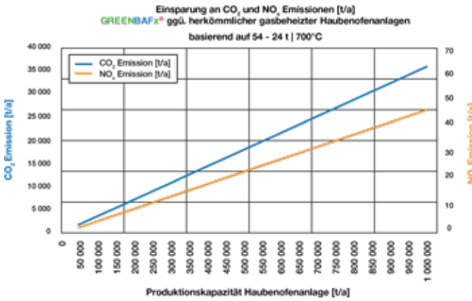
Bild 5: Einsparpotential CO 2 und NO x
