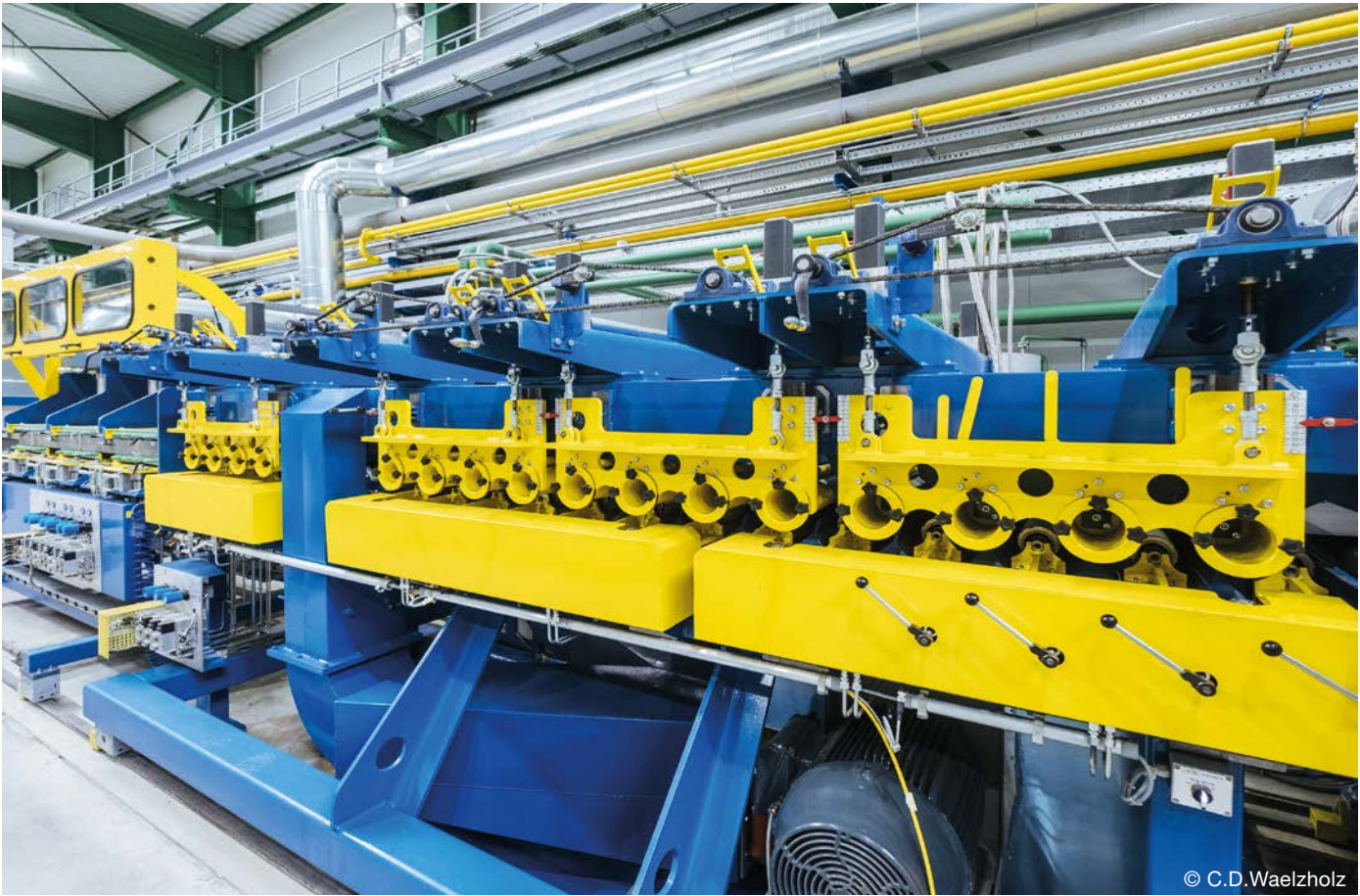
马氏体冷却段
