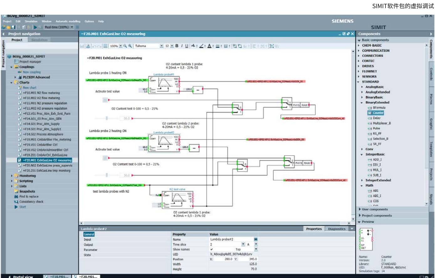
SIMIT软件包的虚拟调试
