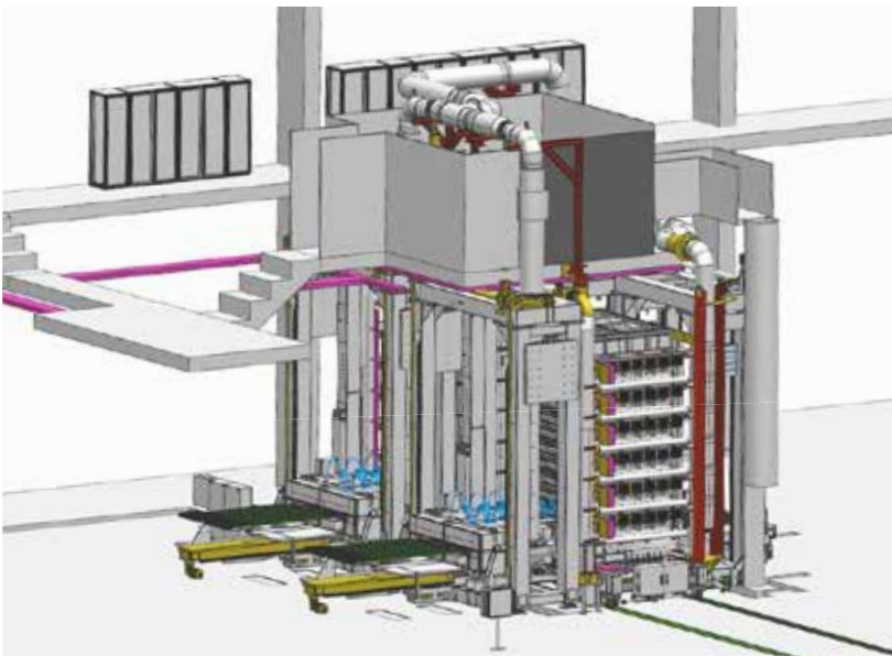
多层批式炉用于局部硬化。
